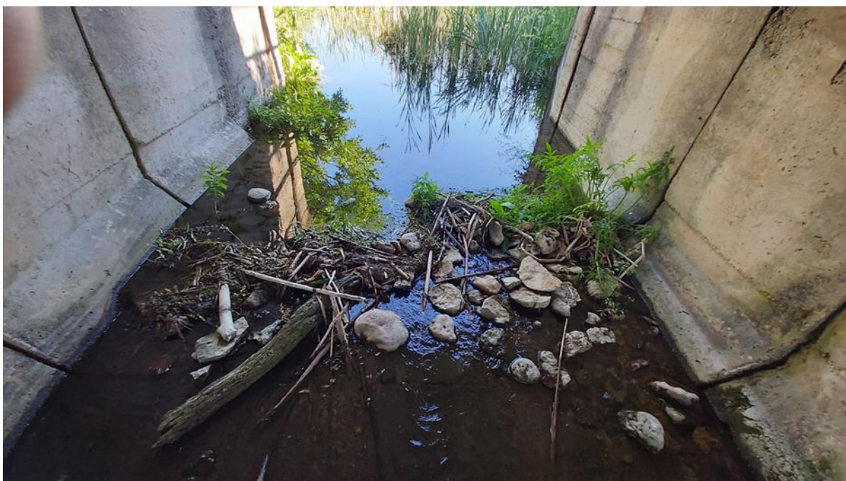
Foto 4. Risu sissevoolu põhjas, mis madala veeseisu korral võib takistada kalade liikumist (25.06.2020)
